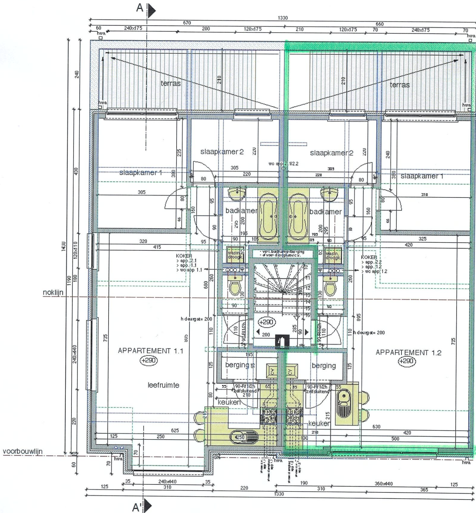
VERDIEPING 01 - schaal 1/50
