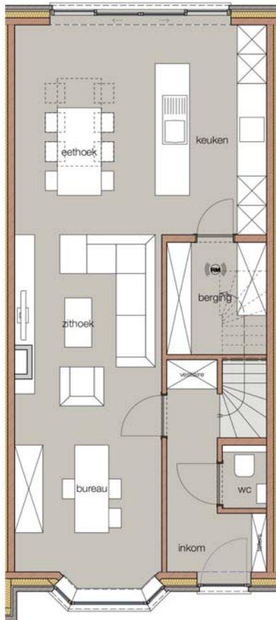
Gelijkvloers
