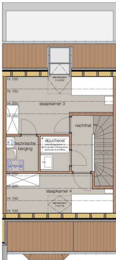
Tweede verdieping
