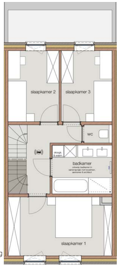
Eerste verdieping
