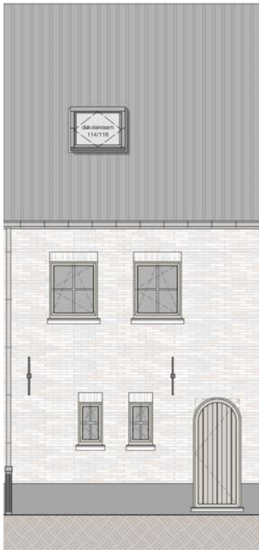
Voorgevel
