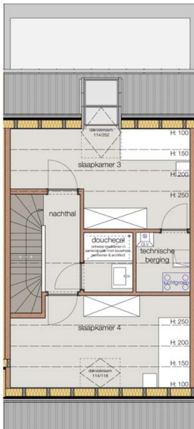
Tweede verdieping
