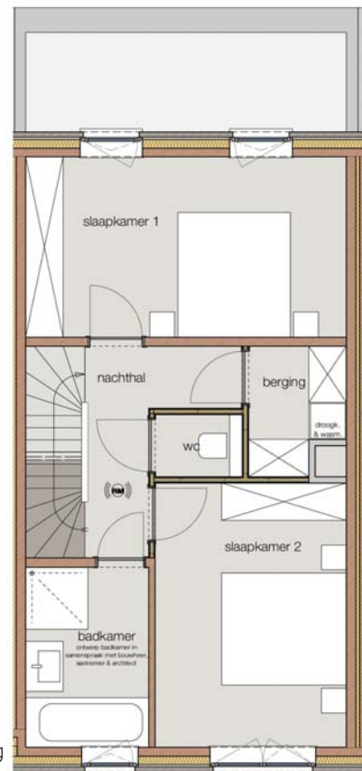
Eerste verdieping
