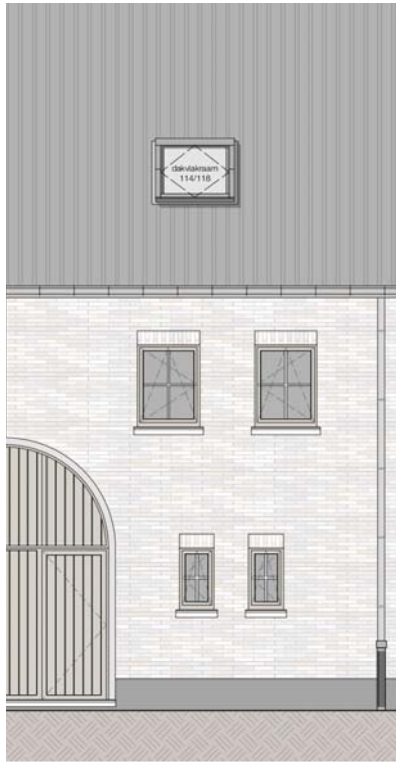
Voorgevel
